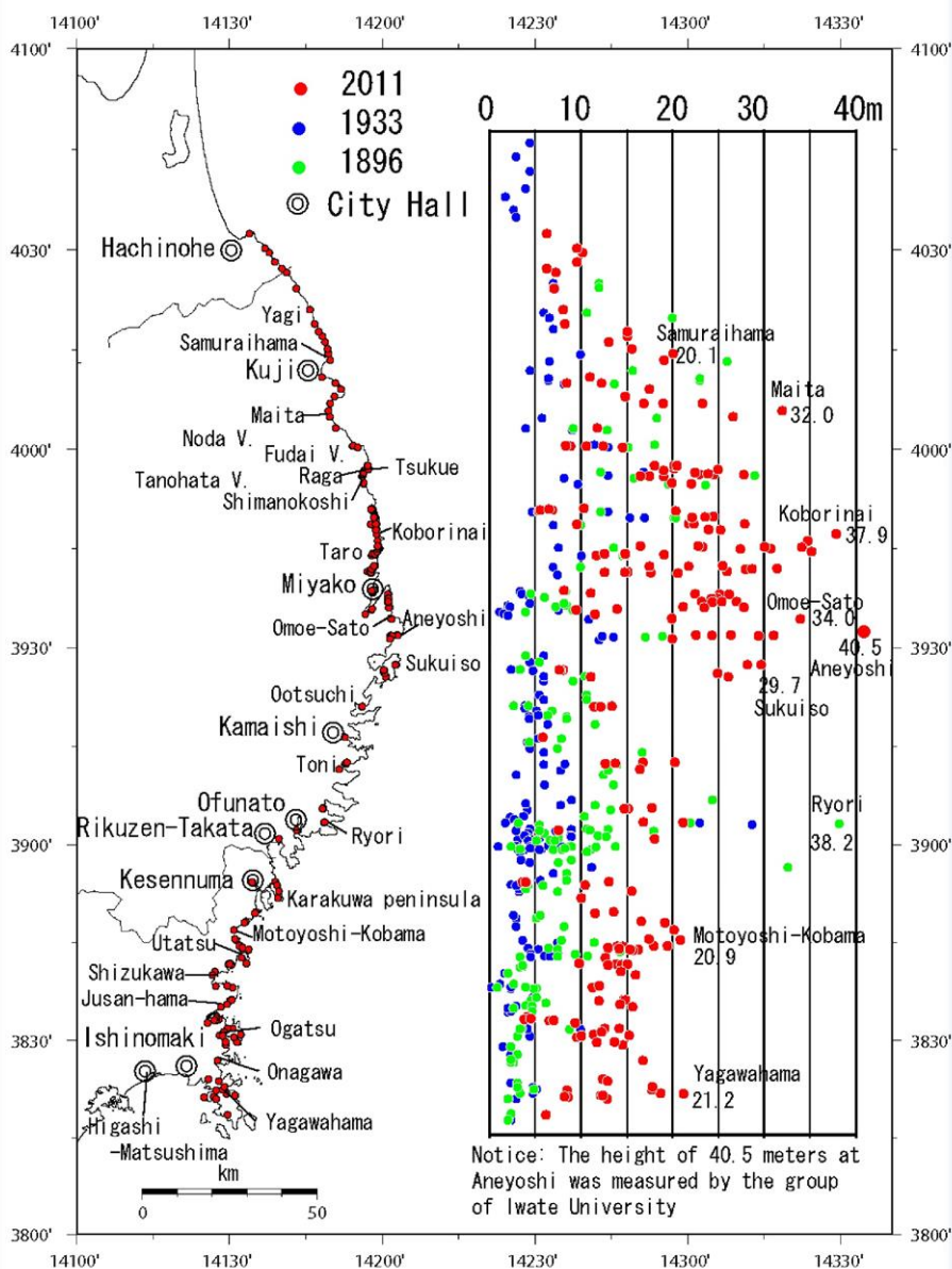
東北地方太平洋沿岸域を襲った津波高分布図
